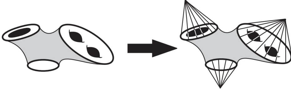
Fig. 1.10. Singular manifold
